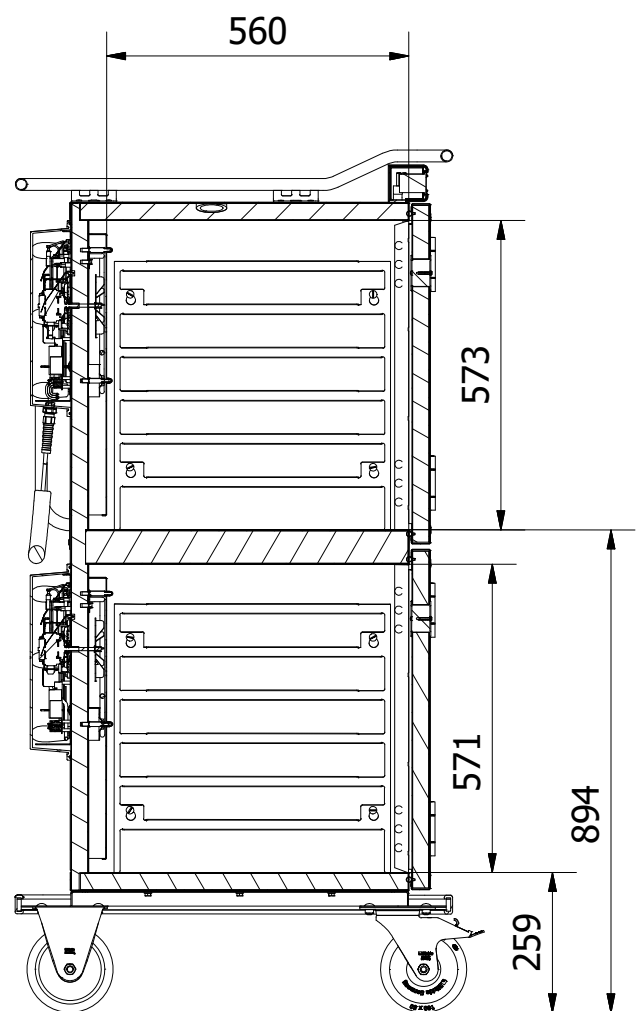
A-A ( 1:14 )
